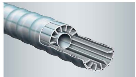
Mehrschalige Konvektionsheizfläche
